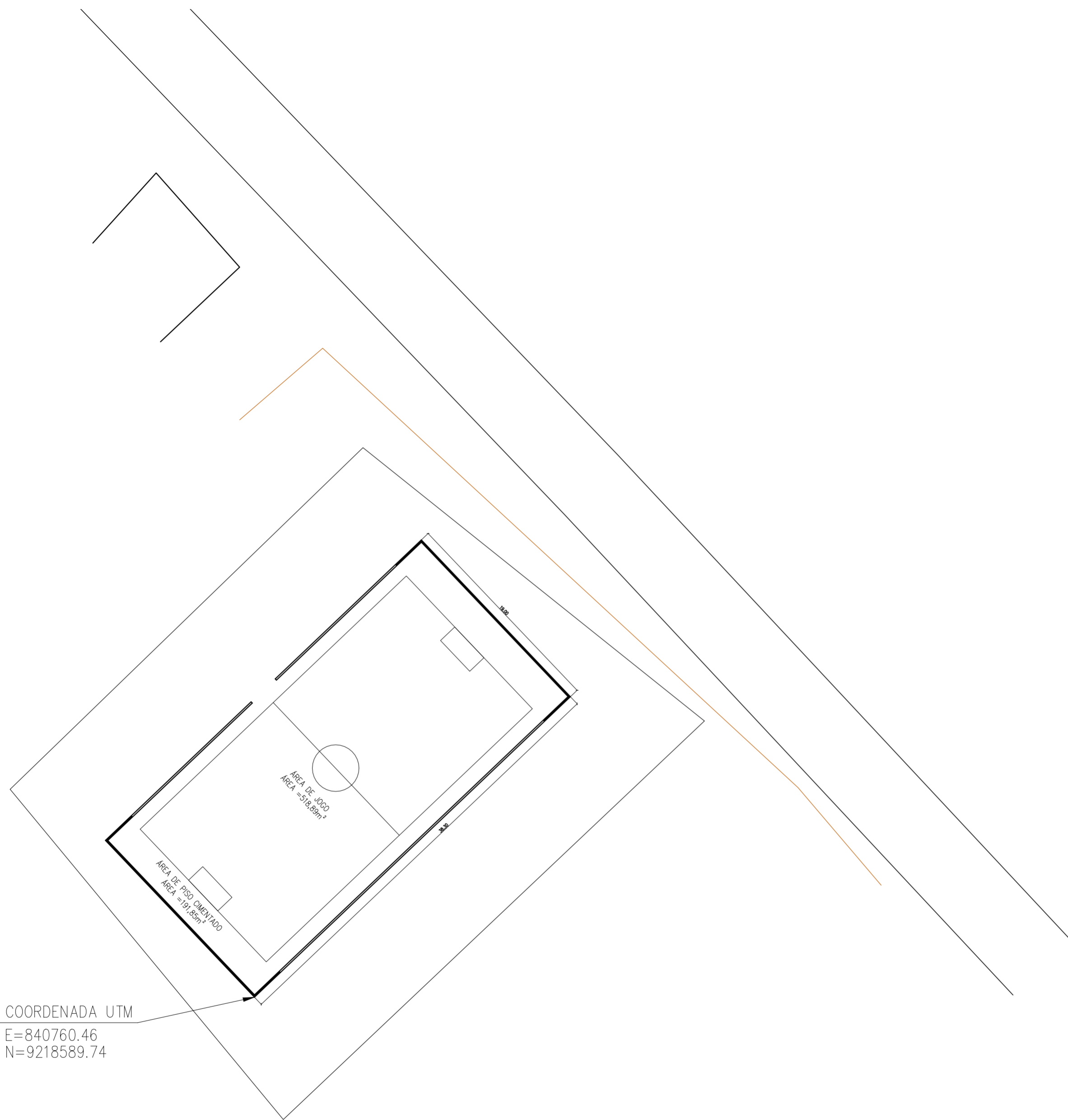
PLANTA DE SITUAÇÃO E LOCAÇÃO LOCALIDADE DIVISÃO ESCALA 1/300
