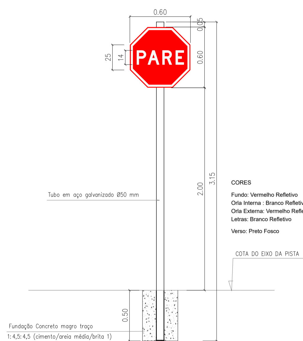
PLACA DE REGULAMENTAÇÃO - L=60cm PARADA OBRIGATORIA - R1 MEDIDAS EM cm
