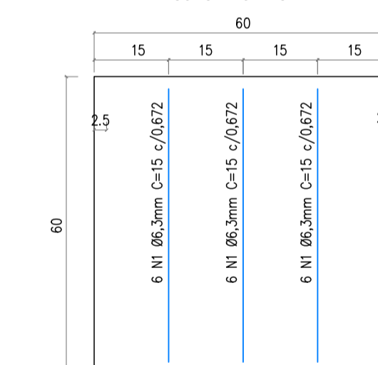
PLANTA BAIXA ESCALA: 1/10
