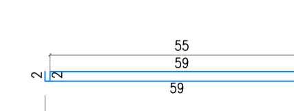
DETALHE TRANSVERSAL DA ARMAÇÃO DA TAMPA DE CONCRETO DA CANALETA ESCALA: 1/10
