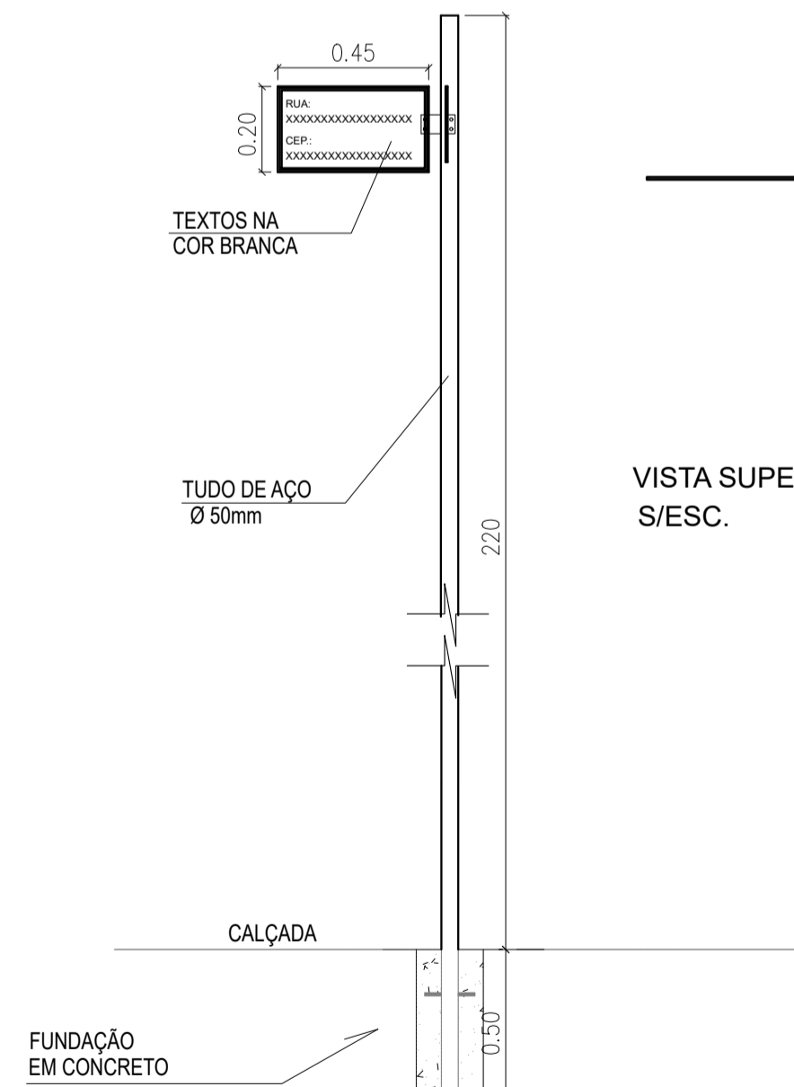
DETALHAMENTO DA PLACA PARA CRUZAMENTOS DE RUA VISTA FRONTAL DA PLACA ESCALA 1/20
