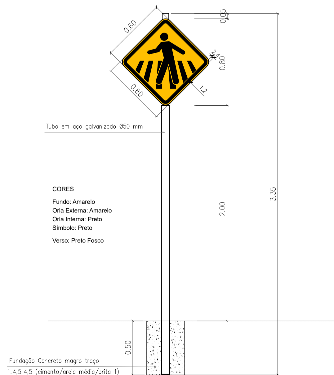
PLACA DE ADVERTÊNCIA - 60x60cm PASSAGEM SINHALIZADA DE PEDESTRES - A32-b MEDIDAS EM cm ESCALA 1/20
